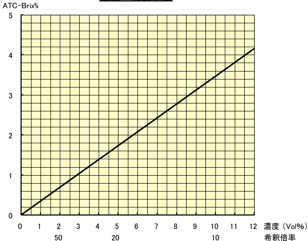
濃度－精度線図
